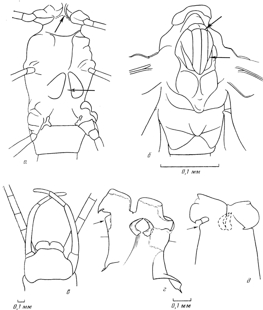
Рис. 1. Heptagenia (Kageronia) fuscogrisea (Retzius); а – г – экз. № Ar. 8984, а – грудь вентрально; б – грудь дорсально (стрелками отмечены признаки, указанные в диагнозе рода); в – гениталии вентрально; г – пенис дорсально (большая часть дорсальной стенки разрушена, видны титилляторы); Калининград; верхний эоцен; д – пенис дорсально; Ленинградская обл.; современный
