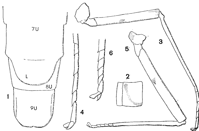
Fig. II. Rhithrogena aurantiaca BURM. Immagine ♀. 1. Estremità posteriore dell'addome veduta ventralmente. 2. Quarto urite visto lateralmente. 3. Zampa anteriore. 4. Tarsolo della stessa. 5. Zampa posteriore. 6. Tarsolo della stessa: L, lamina subgenitale; 7U, 8U, 9U, settimo, ottavo e nono urotergite.
