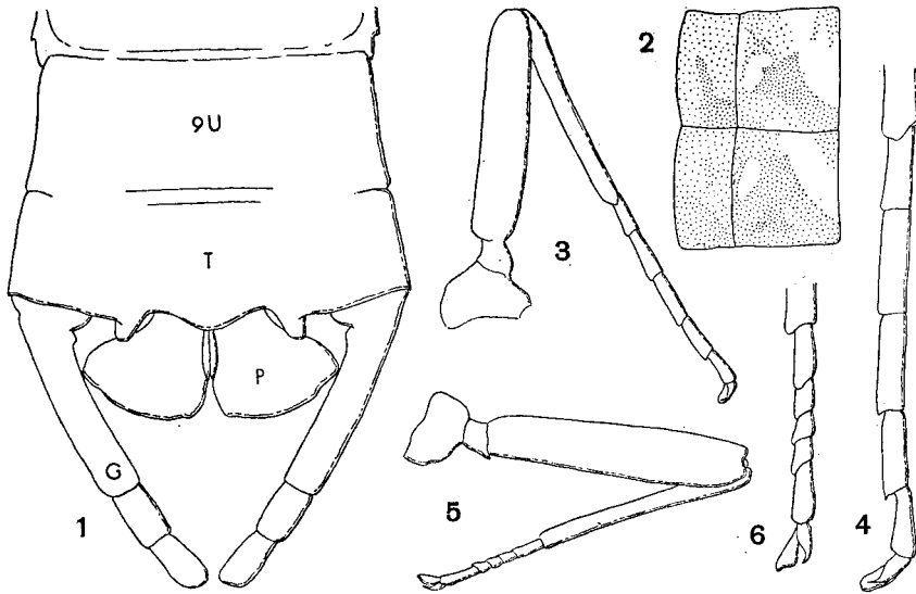
Fig. III. Ecdyonurus venosus F. Subimmagine ♂. 1. Nono urosterno e organi copulatori veduti ventralmente. 2. Terzo e quarto urite visti lateralmente. 3. Zampa anteriore. 4. Tarso della stessa. 5. Zampa posteriore. 6. Tarso della stessa: G. gonostili; P, peni; T, stiligero; 9U, nono urosterno.
