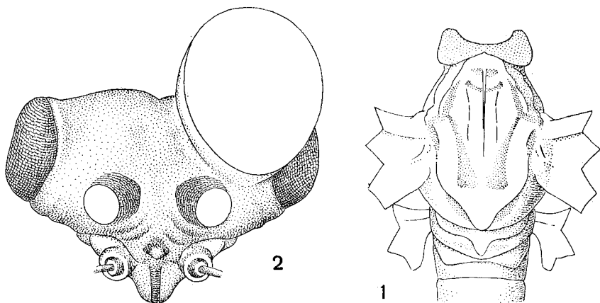
Fig. IV. 1. Ecdyonurus venosus F., subimmagine ♂, torace visto dorsalmente. 2. Baëtis sp., immagine di individuo ginandromorfo, capo visto anteriormente.
