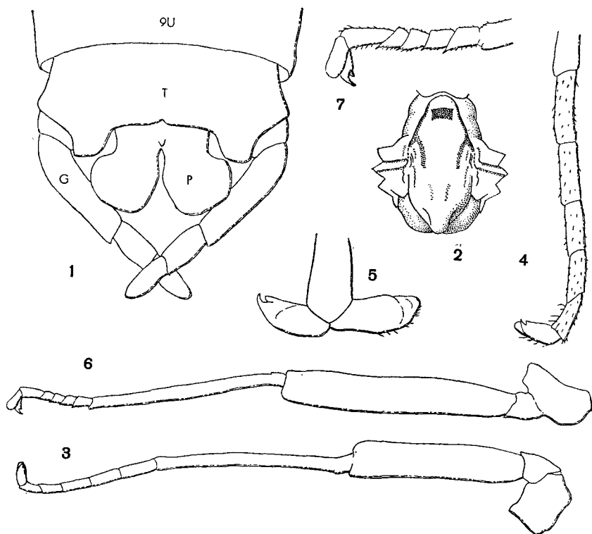
Fig. 1. Epeorus assimilis ETN. Subimmagine ♂. 1. Parte del nono urosterno e organi copulatori veduti ventralmente. 2. Mesotorace veduto dal dorso. 3. Zampa anteriore. 4. Tarsolo della stessa. 5. Estremità distale della stessa. 6. Zampa posteriore. 7. Tarsolo della stessa: G, gonostili; P, peni; T, stiligero; 9U, nono urosterno.
