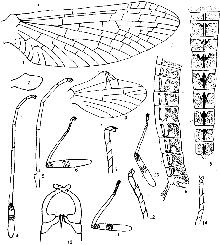
图 1-4 安徽宽基蜉, 新种 Choroterpes (Euthraulius) anhuiensis sp. nov.
