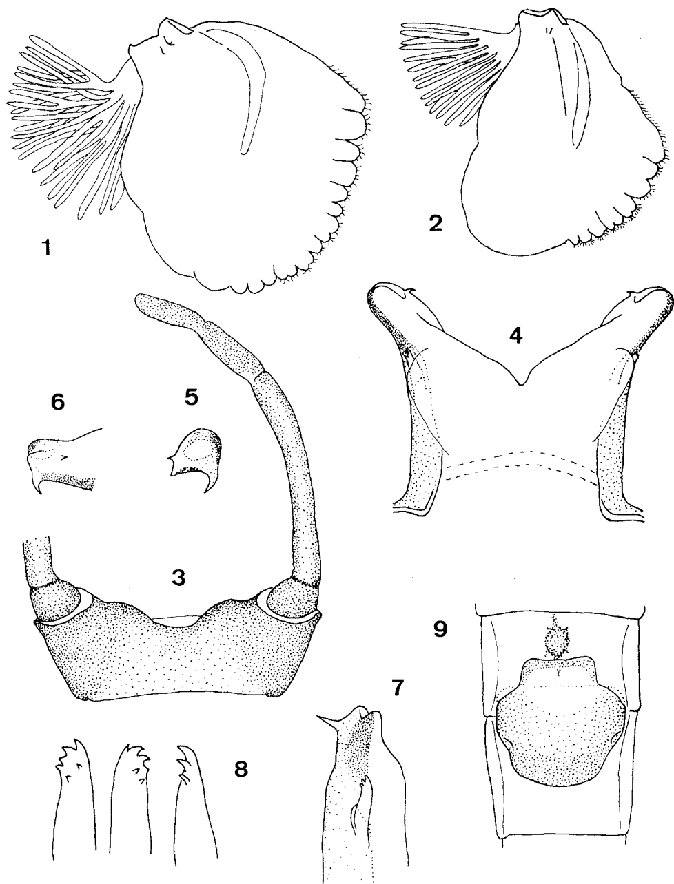
Figs 1—9. Rhithrogena degrangei Sowa, larve du dernier stade (1 et 2) et R. diensis sp. n., imago mâle (3 à 8) et imago femelle (9). 1 — deuxième branchie, côté droit; 2 — sixième branchie; 3 — styligère et gonopodes; 4 — pénis, vue ventrale; 5 — apex du lobe pénien droit, vue apicale; 6 — lobe pénien extrémité distale, vue latéro-interne; 7 — lobe pénien, vue latérale; 8 — titillateurs; 9 — plaque sous-génitale
