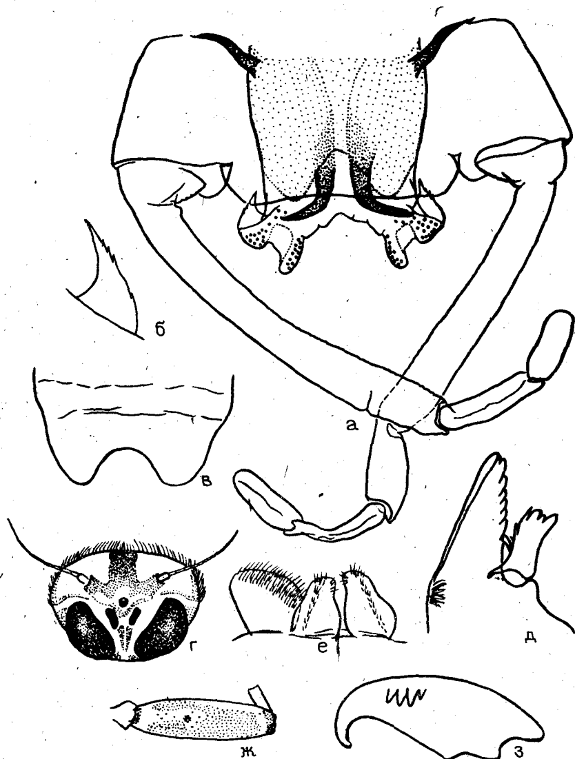
Рис. 4. Детали строения Iron levanidovae Sinitshenkova, sp. n.: а-б — гениталии имаго самца: а — стилитер и пенис, б — зубец на вершине лопасти пениса, преп. № 436; в — постгенитальная пластинка имаго самки, преп. № 438; г-з — детали строения личинки, преп. № 424: г — голова, д — зубцы на вершине левой мандибулы, е — нижняя губа, ж — переднее бедро, з — коготок. Южное Приморье, р. Кедровая
