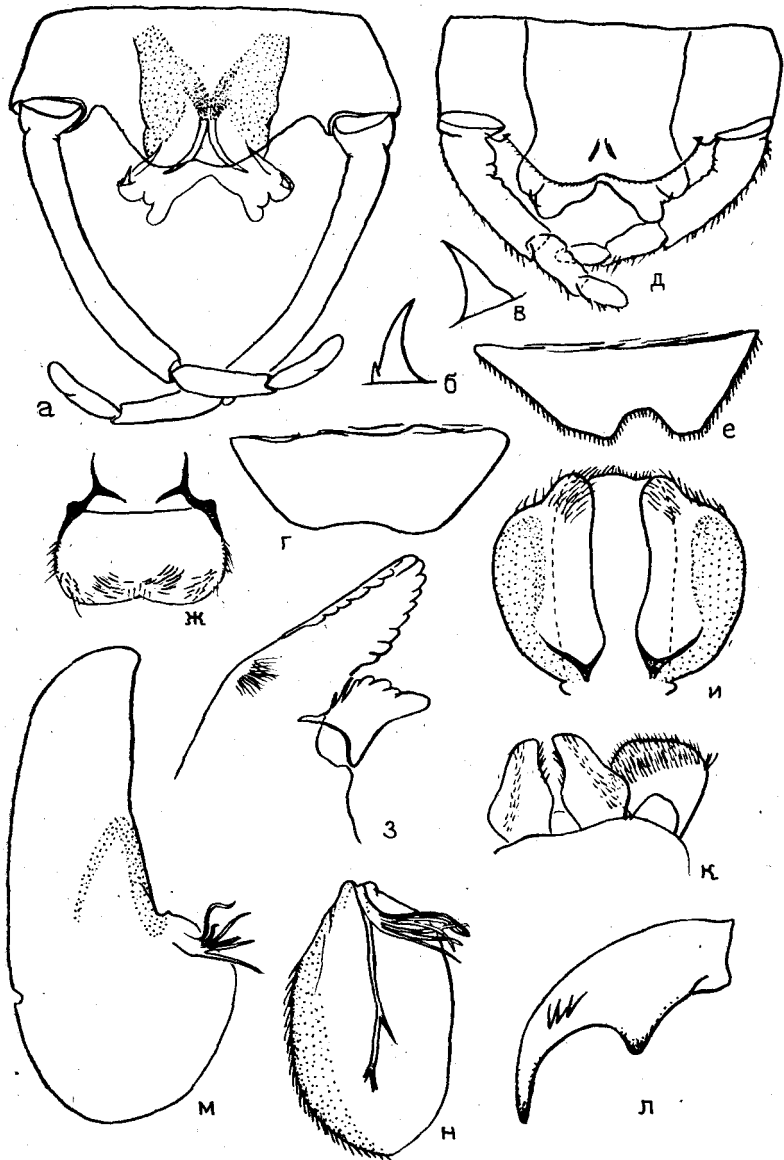
Рис. 1. Детали строения Iron latericius Sinitshenkova, sp. n.: а—в — гениталии имаго самца: а — стилегер и пенис, б, в — зубцы на вершине лопастей пениса, преп. № 426; г — постгенитальная пластинка самки, преп. № 443; д — гениталии субимаго самки, преп. № 449; ж—л — детали строения личинки: ж — верхняя губа, з — зубцы на вершине левой мандибулы, и — гипофаринкс, к — глоссы и паратглоссы нижней губы, л — коготок; м — I жабра; н — V жабра, преп. № 451. Камчатка, р. Кирпичная
