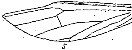
Fig. 79. — Haplosetina tenella NAV., Alle postérieure.
