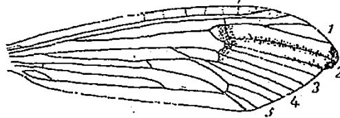
Fig. 76. — Polymorphanisus Elisabethae ♂ NAV. Ala antérieure.
