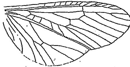
Fig. 71. — Neoperla lujana ♀ NAV. Aile postérieure.
