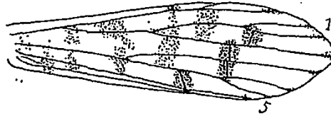
Fig. 78. — Cecetis Hulstaerti NAV. Aile antérieure.
