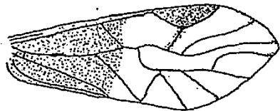
Fig. 69. — Rosega picta NAV. Ala antérieure.
