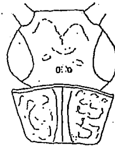
Fig. 72. — Neoperla luluana ♀ NAV. Tête et prothorax.
