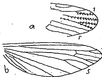
Fig 77. — Homel'a aurifera NAV. a) Bout de l'aile antérieure. b) Aile postérieure.
