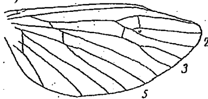
Fig. 74. — Hydropsychodes burgeonia ♀ NAV.. Aile postérieure.
