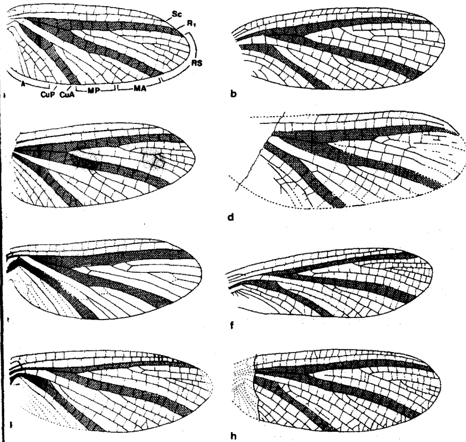
Abb. 1. Die Flügel der bisher beschriebenen Arten der Gattung Misthodotes . a. M. edmundsi (b) M. sharovi b. M. biguttatus (d) M. stapfi n. sp. c. M. delicatulus (f) M. obtusus d. M. ovalis (h) M. zelesskyi
