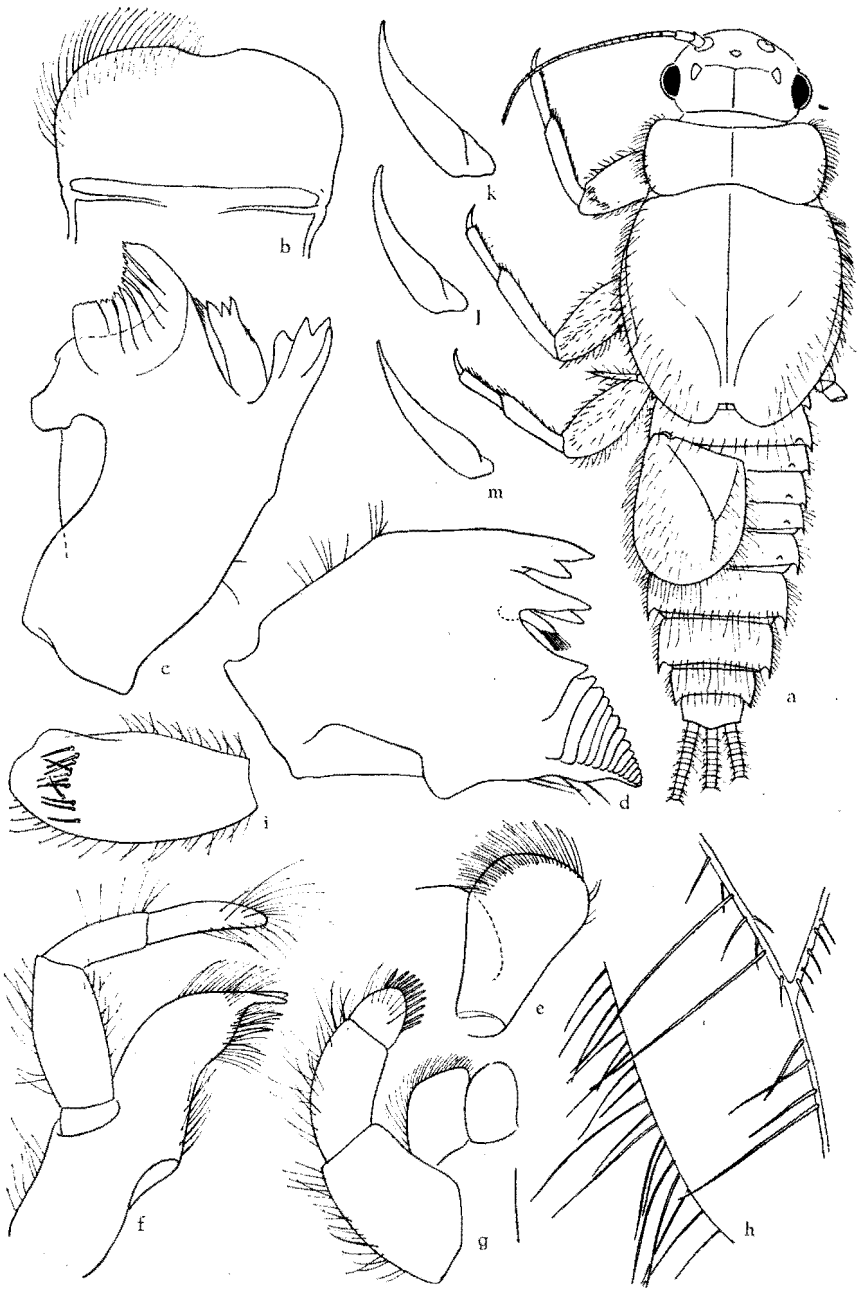
Fig. 14. — Caenodes sp. n° 1, larve.
