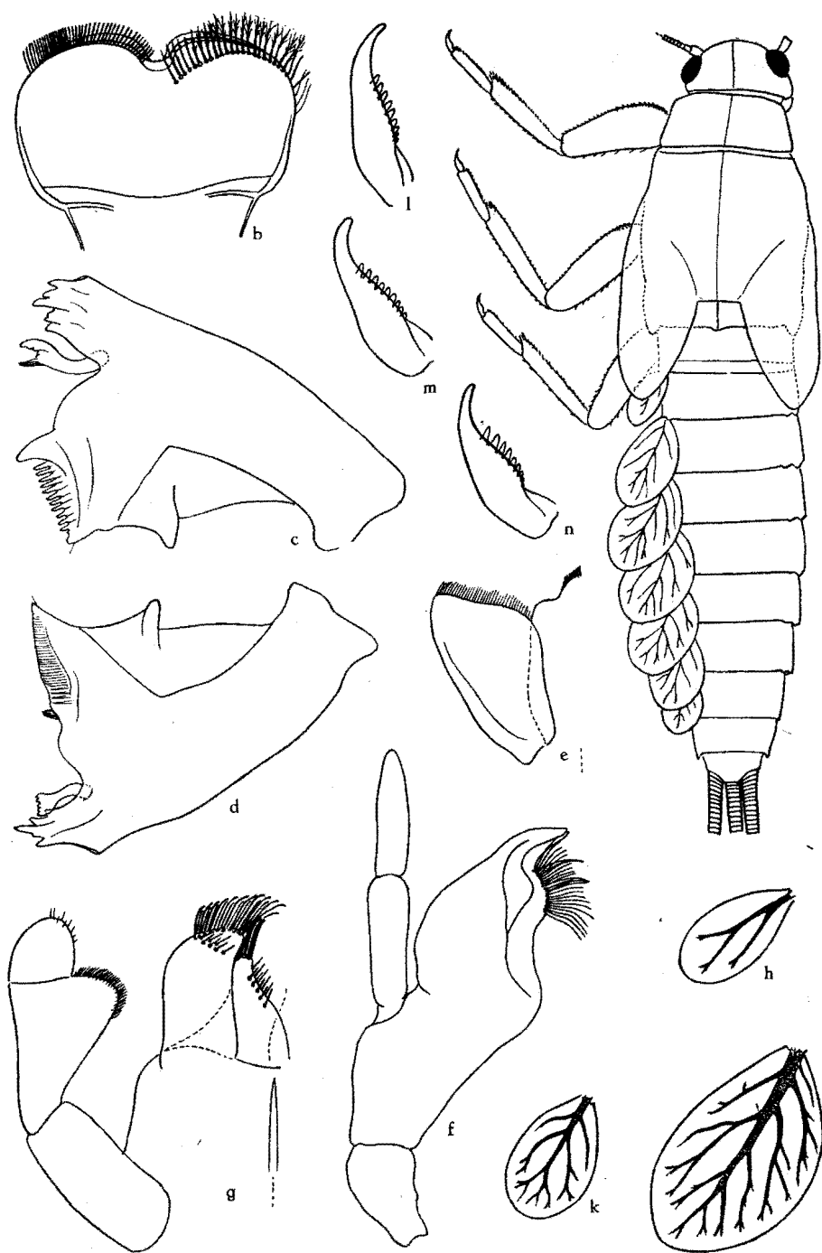
Fig. 1. — Baetis sp. n° 1, larve. a) Vue générale; x 14. b) Labre; x 56. c) Mandibule gauche; x 56. d) Mandibule droite; x 56. e) Hypopharynx; x 56. f) Maxille droite; x 56. g) Labium; x 56. h, i, k) Trachéobranchies I, IV et VII; x 57.5. l, m, n) Ongles I, II et III; x 100.
