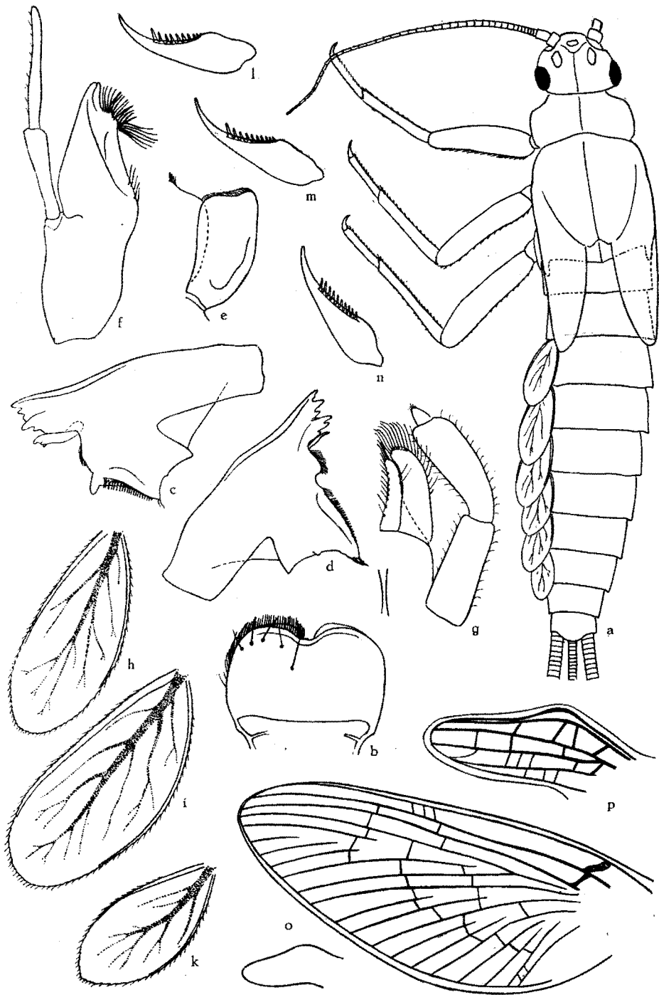
Fig. 7. — Centroptilum sp. n° 1, larve. a) Vue générale; x 14. b) Labre; x 65. c) Mandibule gauche; x 65. d) Mandibule droite; x 65. e) Hypopharynx; x 65. f) Maxille droite; x 65. g) Labium; x 65. h, i, k) Trachéobranchies II, IV et VII; x 45. l, m, n) Ongles I, II et III; x 110. o) Ptérothèques I (contour) et II (contour); x 32. p) Ptérothèque II (nervation); x 70.
