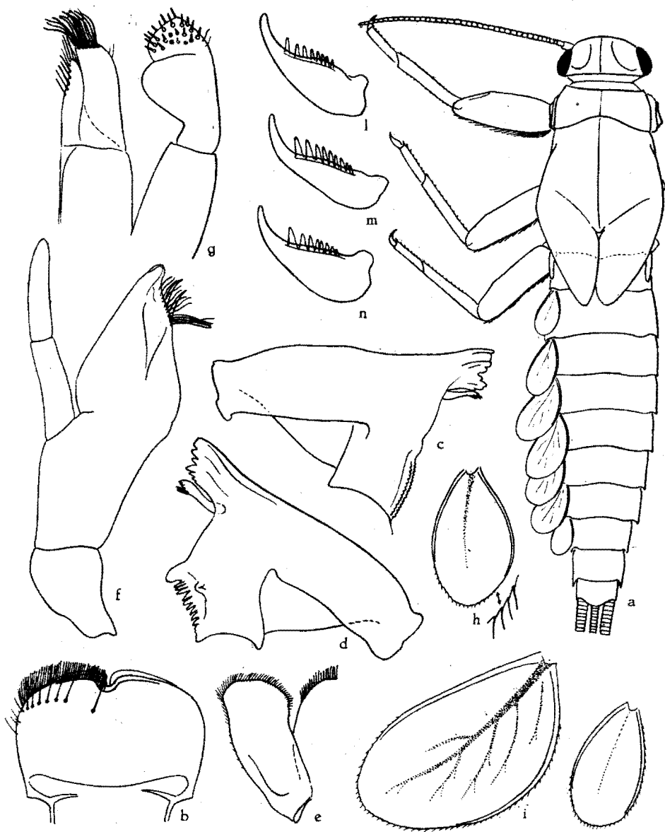
Fig. 2. — Baetis sp. n° 2, larve.
