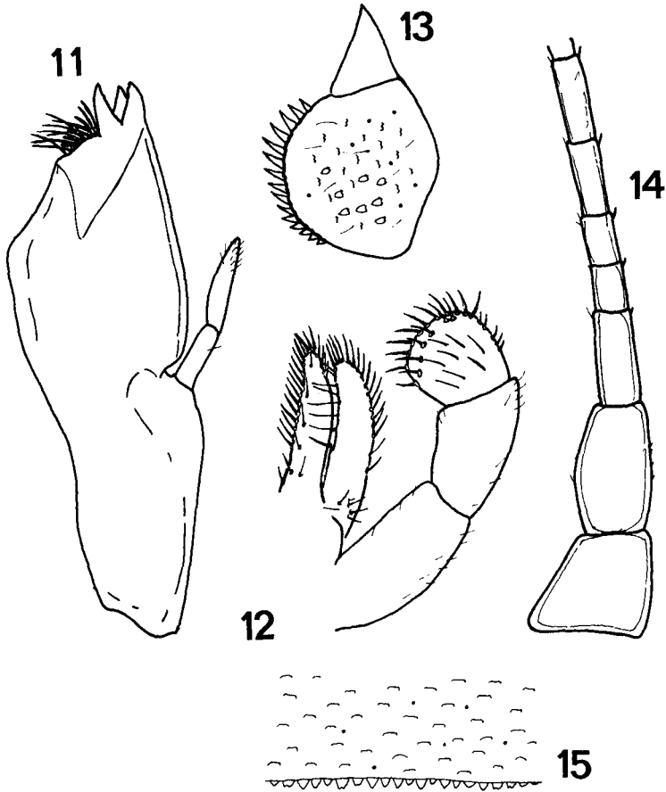
Fig. 11–15. Centroptella longisetosa n. sp., Larve. 11: Maxille mit Palpus – 12: Labium mit Glossa, Paraglossa und Palpus – 13: Paraproct – 14: Fühler – 15: Hinterrand des Tergit III.
