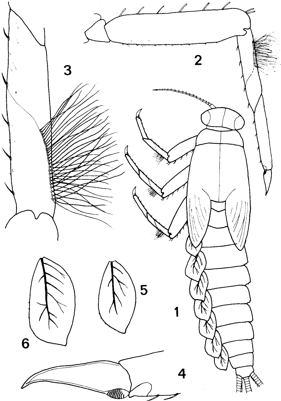
Fig. 1-6. Centropptella longisetosa n. sp., Larve. 1: Gesamtansicht - 2: Vorderbein - 3: Tibia mit Borstensaum - 4: Kralle - 5: Kieme I - 6: Kieme III
