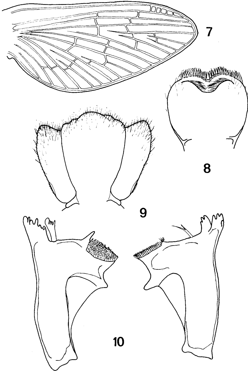
Fig. 7-10. Centroptella longisetosa n. sp., Larve. 7: Vorderflügel (aus der Larve herauspräpariert) - 8: Labrum - 9: Hypopharynx - 10: Mandibeln.
