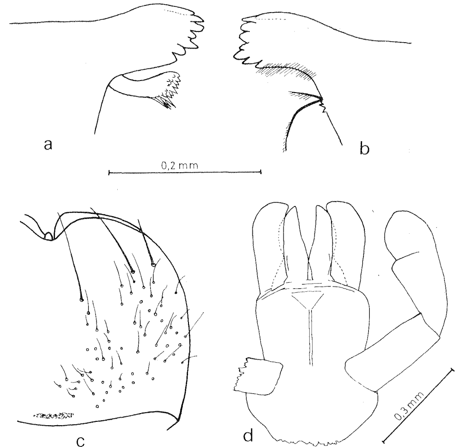
Fig. 1.—Piezas bucales de Baetis muticus intermedius nov. ssp.: a) región incisiva de la mandíbula izquierda; b) ídem de la mandíbula derecha; c) superficie externa del labro; d) configuración general del labro.
