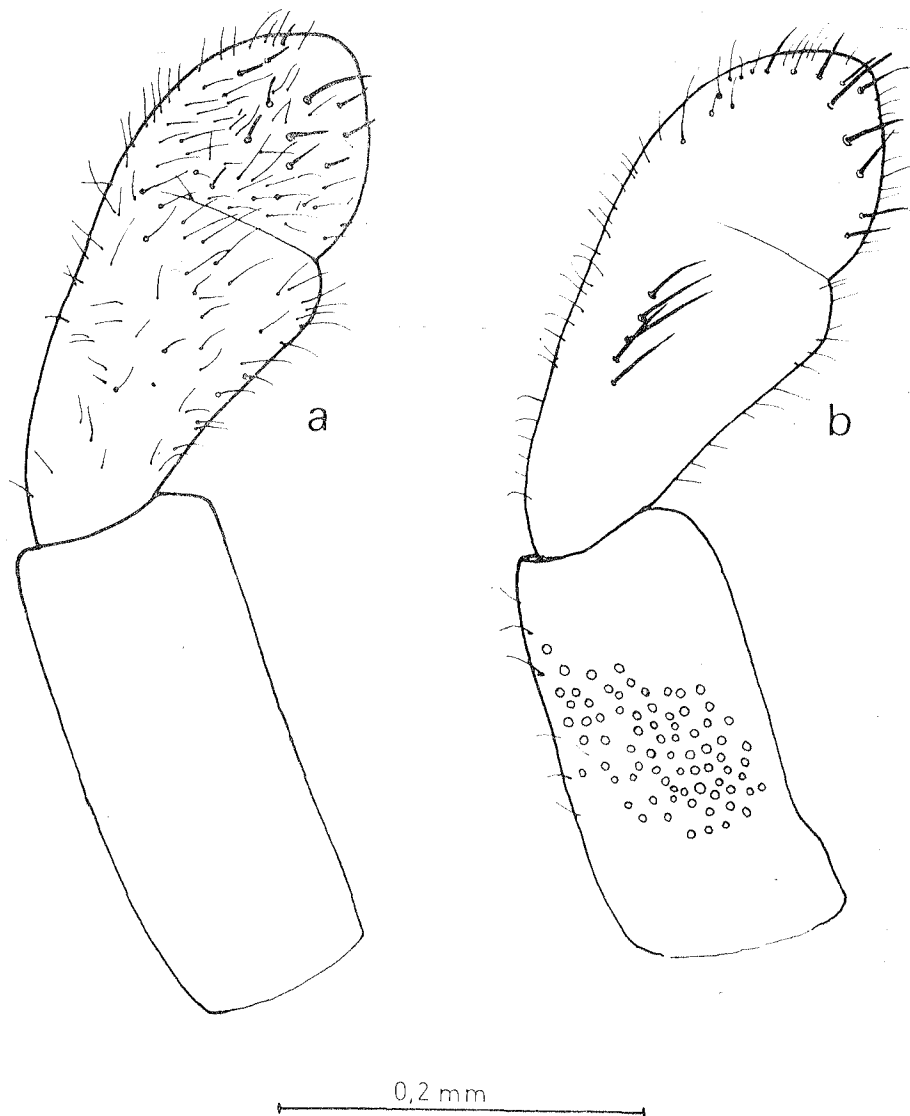
Fig. 2.—Palpo labial de Bactis muticus intermedius nov. ssp.: a) cara inferior; b) cara superior.
