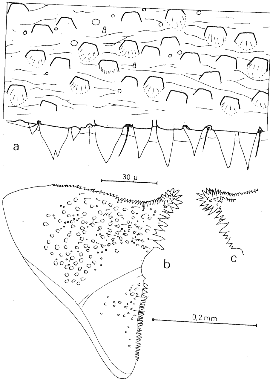
Fig. 3.— Baetis muticus intermedius nov. ssp.: a) superficie y margen posterior de uno de los tergos abdominales medios; b) lámina paraproctal derecha; c) prolongación apical de la lámina paraproctal izquierda.
