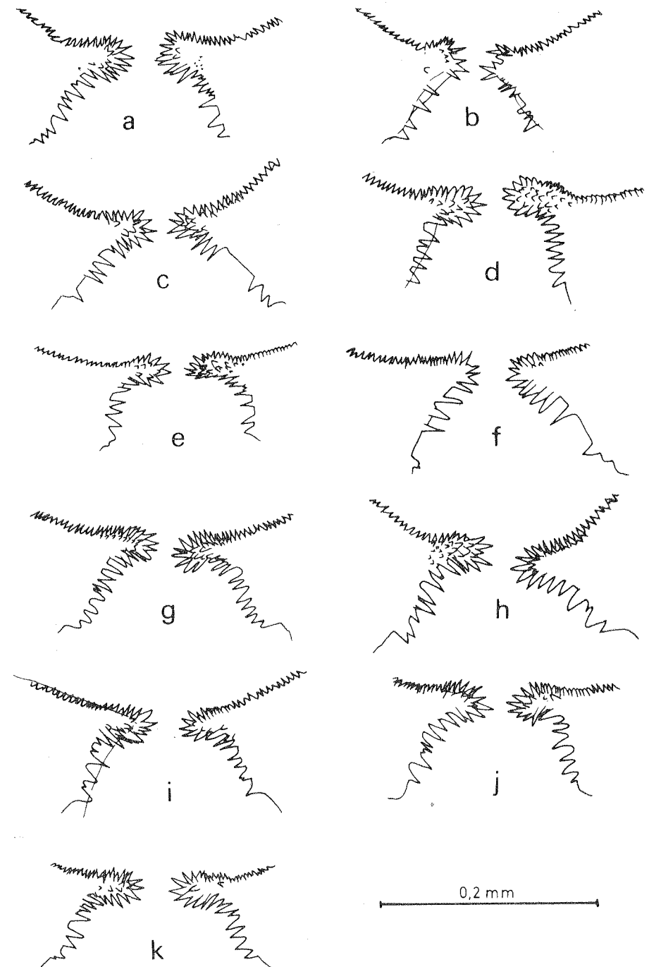
Fig. 4.—Variabilidad que presentan las prolongaciones apicales internas de Baetis muticus intermedius nov. ssp.: a), b), c), d), e), f), g), h), i), j) pertenecen a ejemplares de Sierra Nevada; k) pertenecen a un ejemplar de los Pirineos.
